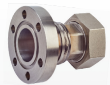
GA-DO-CDH M38x1.5 (P S max: 130 bar)
